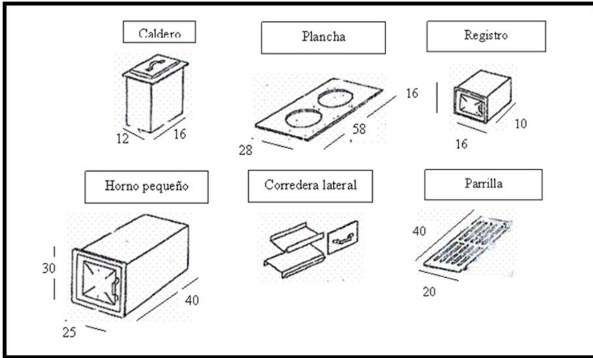
Ilustración 2. Partes componentes de la hornilla eco-eficiente
